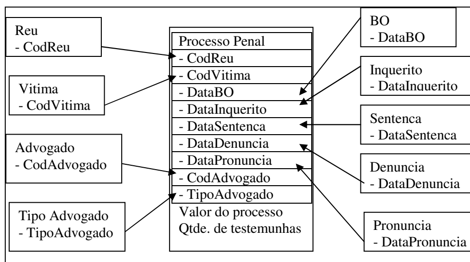
Figura 01 – Modelo Multidimensional
