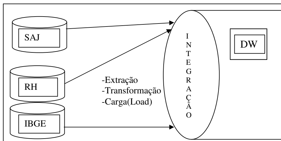
Figura 02 – ETL
