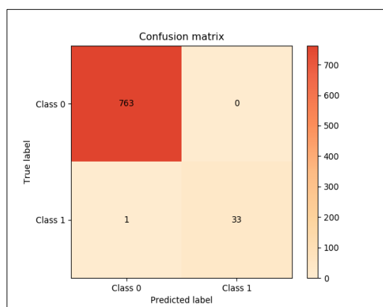
Fig. 6: Matriz de confusión obtenida durante la etapa de prueba por el algoritmo k-Nearest Neighbours con K=1 vecinos cercanos.
